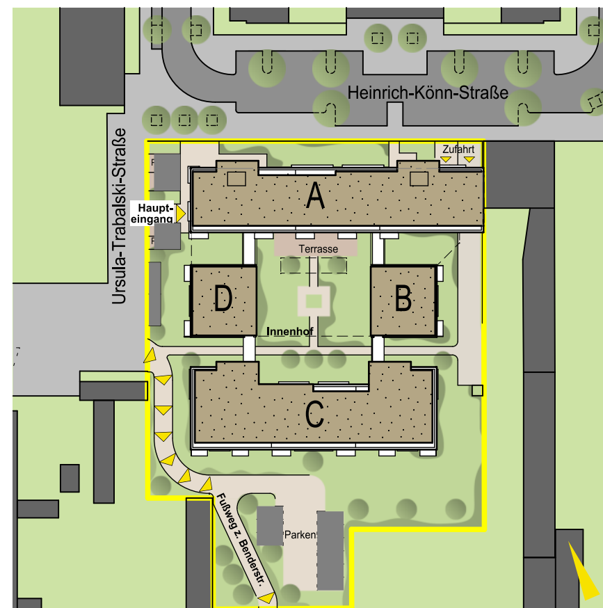
LAGEPLAN
